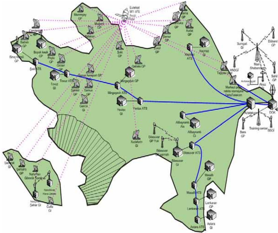
SXEM 1. Azərbaycan Respublikasının gömrük orqanlarında fəaliyyətdə olan qlobal korporativ şəbəkənin funksional sxemi
