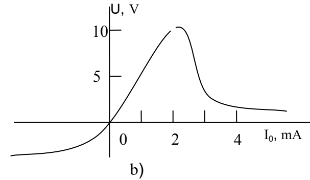
Şəkil 2.1. Kristadinin prinsipial sxemi (a) və VAX-1 (b).
