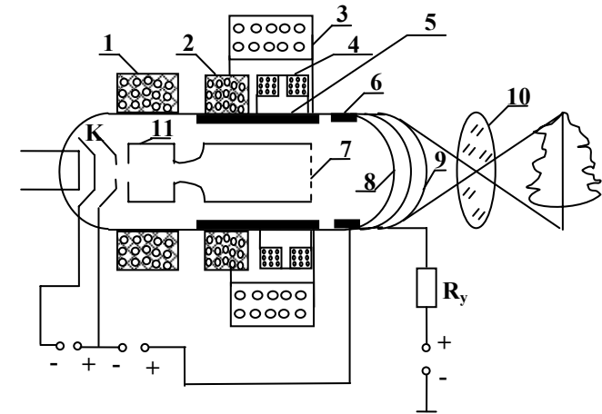
Şəkil 1.7. Vidikonun prinsipial sxemi. 1 – korrektədiçi sarğı, 2 – mərkəzləşdirici sarğı, 3 – fokuslayıcı sarğı, 4 – meyletdirici sarğı, 5, 6 – sürətləndirici anodlar, 7 – tor, 8 – fotorezistor, 9 – siqnal lövhəciyələri, 10 – linza, 11 – idarəedici elektrod
