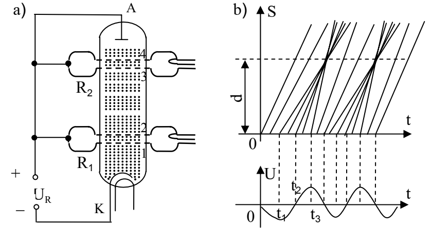
Şəkil 4.1. İkirezonatorlu uçuş klistronunun prinsipli quruluşu (a) və elektron sıxlaşmasının qrafiki təsviri (b)
