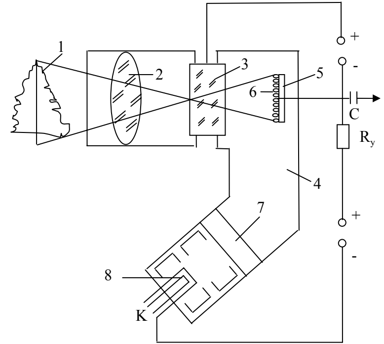
Şəkil 1.6. İkonoskopun prinsipial sxemi. 1 – obyekt, 2 – şəffaf linza, 3 – kollektor, 4 – şüşə balon, 5 – fotokatod, 6 – işıq həssas mozaika, 7 – meyletdirici sistem, 8 – elektron mənbəyi, R_y – yük müqaviməti, C – kondensator.
