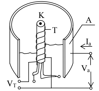
Şəkil 1.2. Triod. A – anod, K – katod, T – tor
