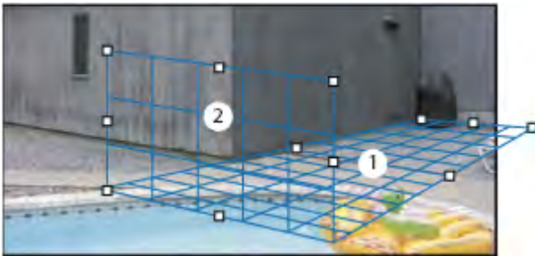
Перекрывающиеся плоскости
