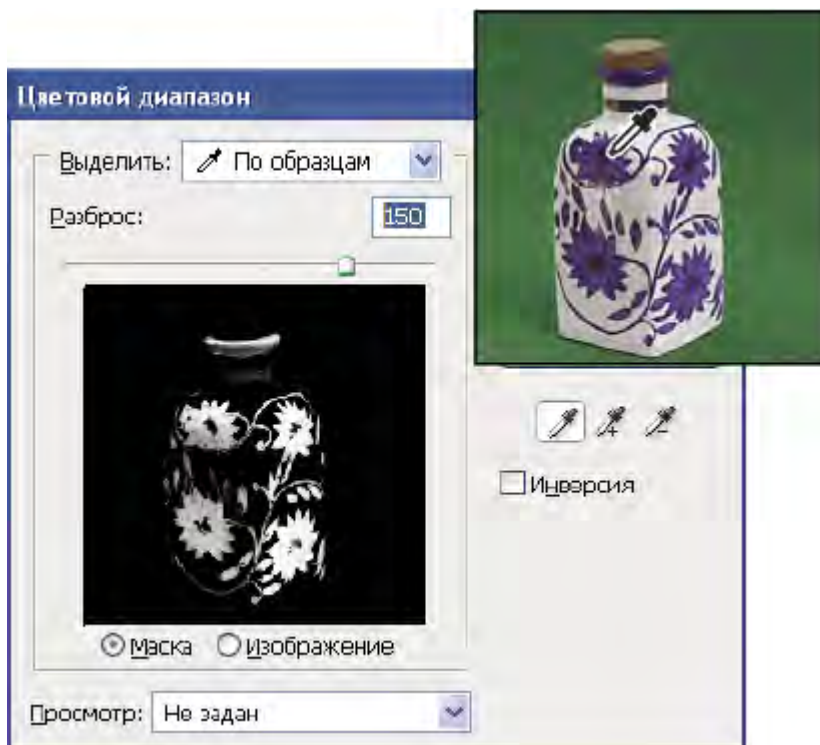
Взятие образца
