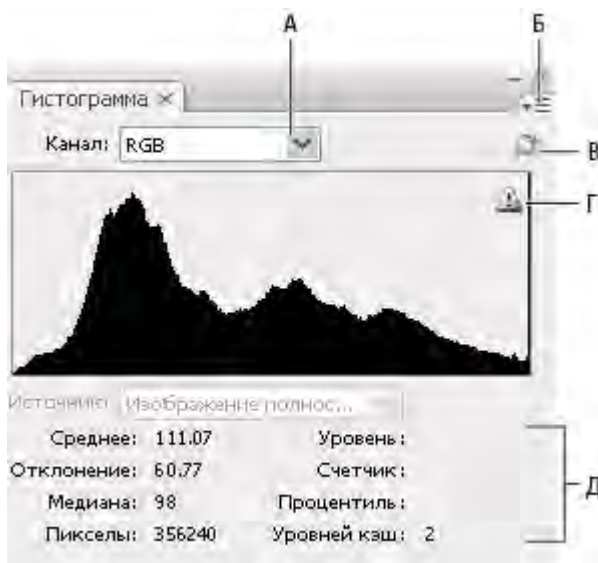
Палитра гистограмм
