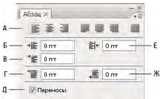
Палитра "Абзац"
