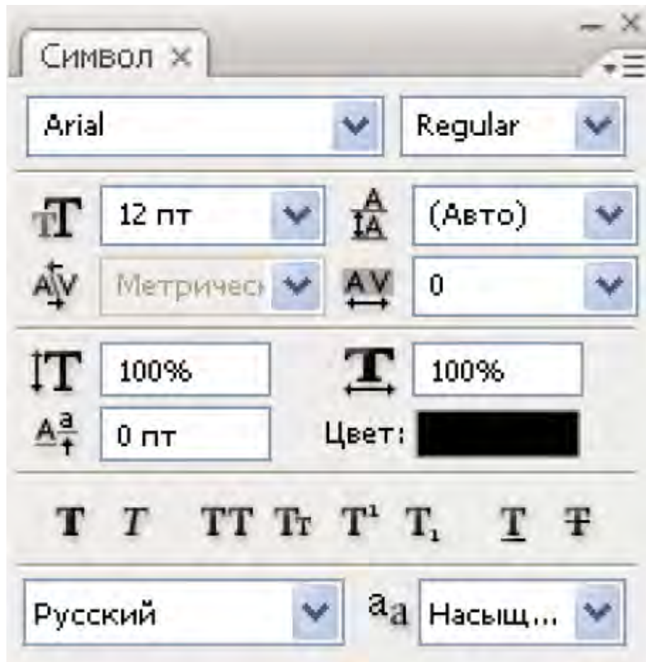
Палитра "Символ"
