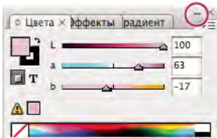
Кнопка "Свернуть"
