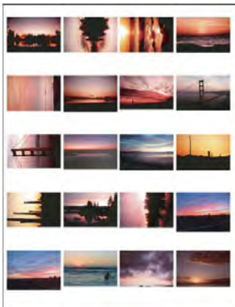
Контрольный лист
