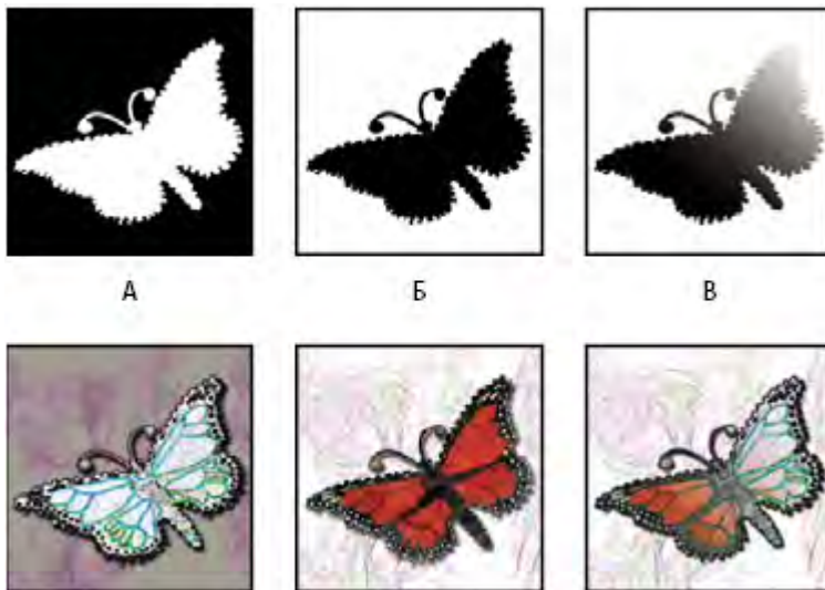
Примеры масок
