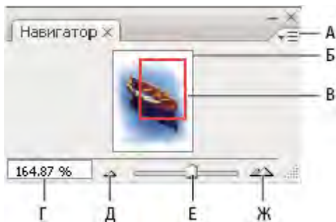
Палитра "Навигатор"
