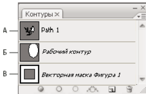
Палитра "Контур"
