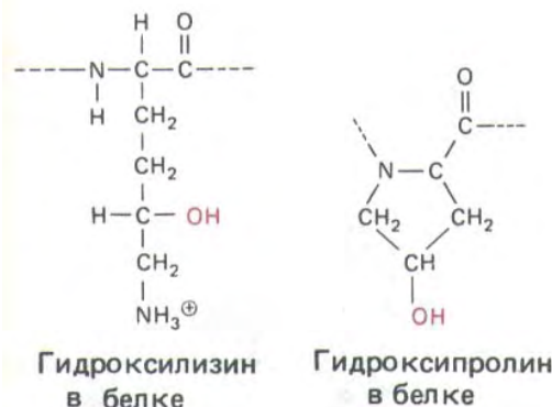
Рис. 14-35. Структура остатков гидроксипролина и гидроксизина - двух измененных аминокислот, обычно содержащихся в коллагене.
