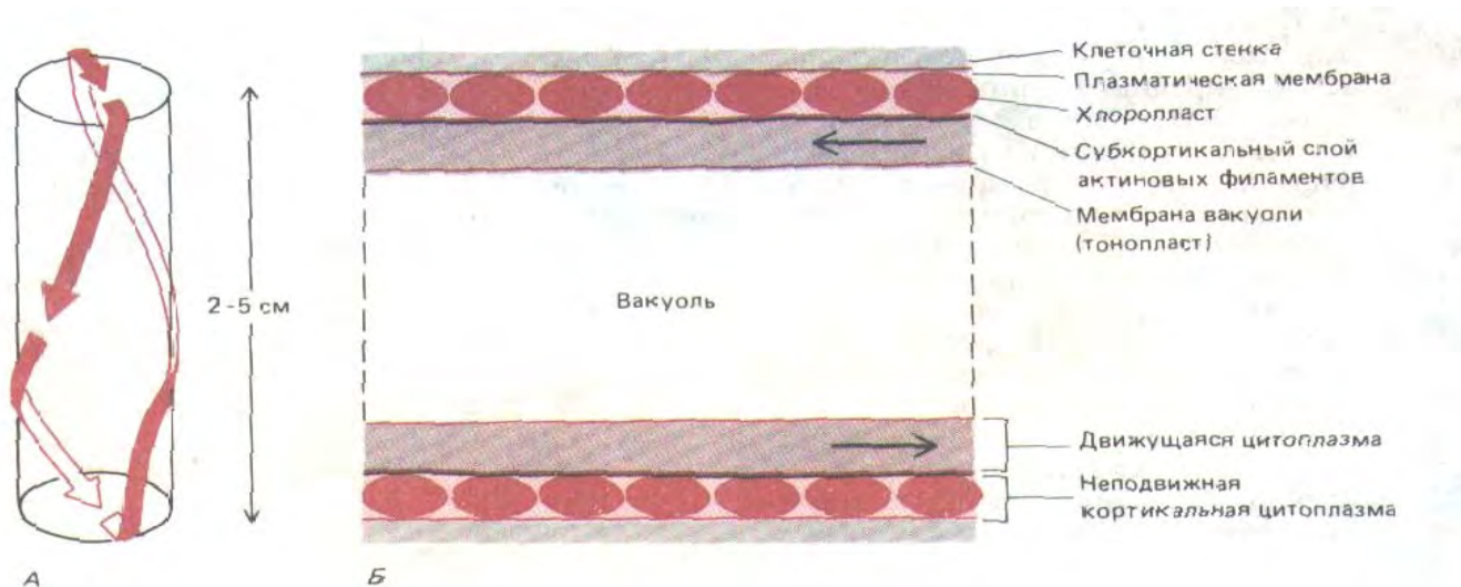
Рис. 11-33. Схема токов цитоплазмы в гигантской клетке водоросли Nitella . А. Путь движения цитоплазмы в цилиндрической клетке. Для простоты диаметр клетки относительно ее длины преувеличен. Б. Продольный разрез участка такой клетки; показана организация неподвижных и движущихся слоев цитоплазмы. В неподвижном кортикальном слое лежат хлоропласты, которые связаны с подлежащими пучками актиновых филаментов; под этими пучками расположен движущийся слой цитоплазмы, в нем находятся ядра, митохондрии и другие органеллы. На самом деле относительные размеры вакуоли гораздо больше, чем на рисунке.
