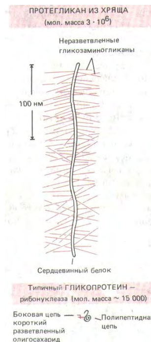
Рис. 14-27. Молекула главного протеогликана хряща. Она состоит из множества гликозаминогликановых цепей, ковалентно связанных с сердцевинным белком. В дополнение к гликозаминогликановым цепям сердцевинный белок содержит еще олигосахаридные цепи, присоединенные к атомам азота или кислорода (на рисунке не показаны). Большинство протеогликианов меньше того, который здесь изображен, и гликозаминогликановые цепи у них часто имеются лишь в определенных областях полипептидной цепи сердцевинного белка. Внизу для сравнения в том же масштабе изображена молекула типичного гликопротеина (панкреатической рибонуклеазы В).
