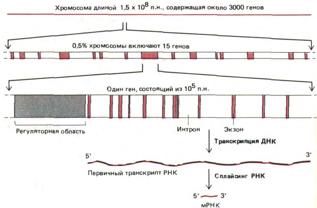
Рис. 9-7. Организация генов в типичной хромосоме позвоночных. Белки, связывающиеся с ДНК в регуляторных областях, определяют транскрипцию гена. Регуляторные последовательности, как правило, расположены на 5'-конце гена (как показано на схеме), но могут находиться в интронах, экзонах и на 3'-конце. При образовании молекул информационной РНК (мРНК) последовательности интронов из первичных транскриптов РНК удаляются. Приведенные здесь данные по количеству генов в хромосоме соответствуют минимальной оценке.
