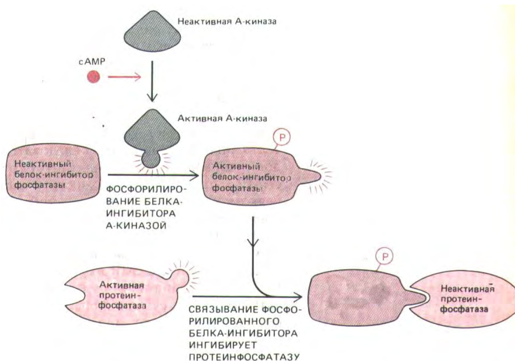
Рис. 12-28. Циклический АМР ингибирует протеинфосфатазу, которая в активном состоянии противодействовала бы реакциям фосфорилирования, запускаемым cAMP. Он активирует А-киназу, а она фосфорилирует белок-ингибитор, который после этого присоединяется к протеинфосфатазе и подавляет ее активность.
