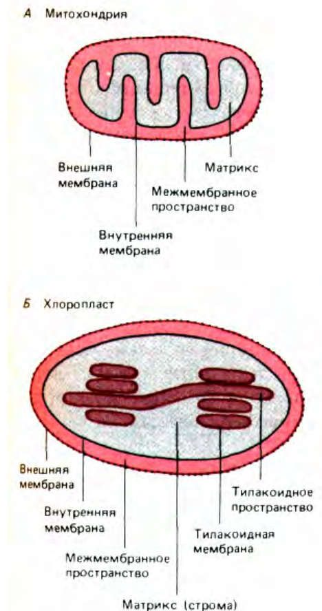
Рис. 8-26. Основные субкомпарменты митохондрий и хлоропластов. Топология хлоропласта может быть получена из топологии митохондрий простым способом: если впячивания внутренней митохондриальной мембраны полностью отпочкуются, то получится компартмент, топологически эквивалентный тилакоидам хлоропластов.
