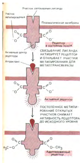
Рис. 12-47. Последовательные процессы активации и адаптации (в результате метилирования) хемотаксического рецептора. Обратите внимание, что активность рецептора (а значит, и частота кувырканий бактерии) в исходном и в адаптированном состоянии одинакова. Для простоты рецептор показан с двумя участками метилирования, в действительности же у каждого рецептора их четыре. При повышении концентрации лиганда доля времени, когда рецептор занят лигандом, увеличивается. Более высокая концентрация лиганда вызывает большее конформационное изменение рецептора, чем низкая, и приближает его состояние к предельно измененному. Однако медленное усиление метилирования через несколько минут восстанавливает исходную конформацию, причем большей концентрации аттрактанта соответствует большее число метильных групп на рецепторе. Рецептор теперь адаптирован. Хотя на схеме показано прямое присоединение лиганда к рецептору, в некоторых случаях он сначала присоединяется к периплазматическому субстрат-связывающему белку, который затем взаимодействует с рецептором.
