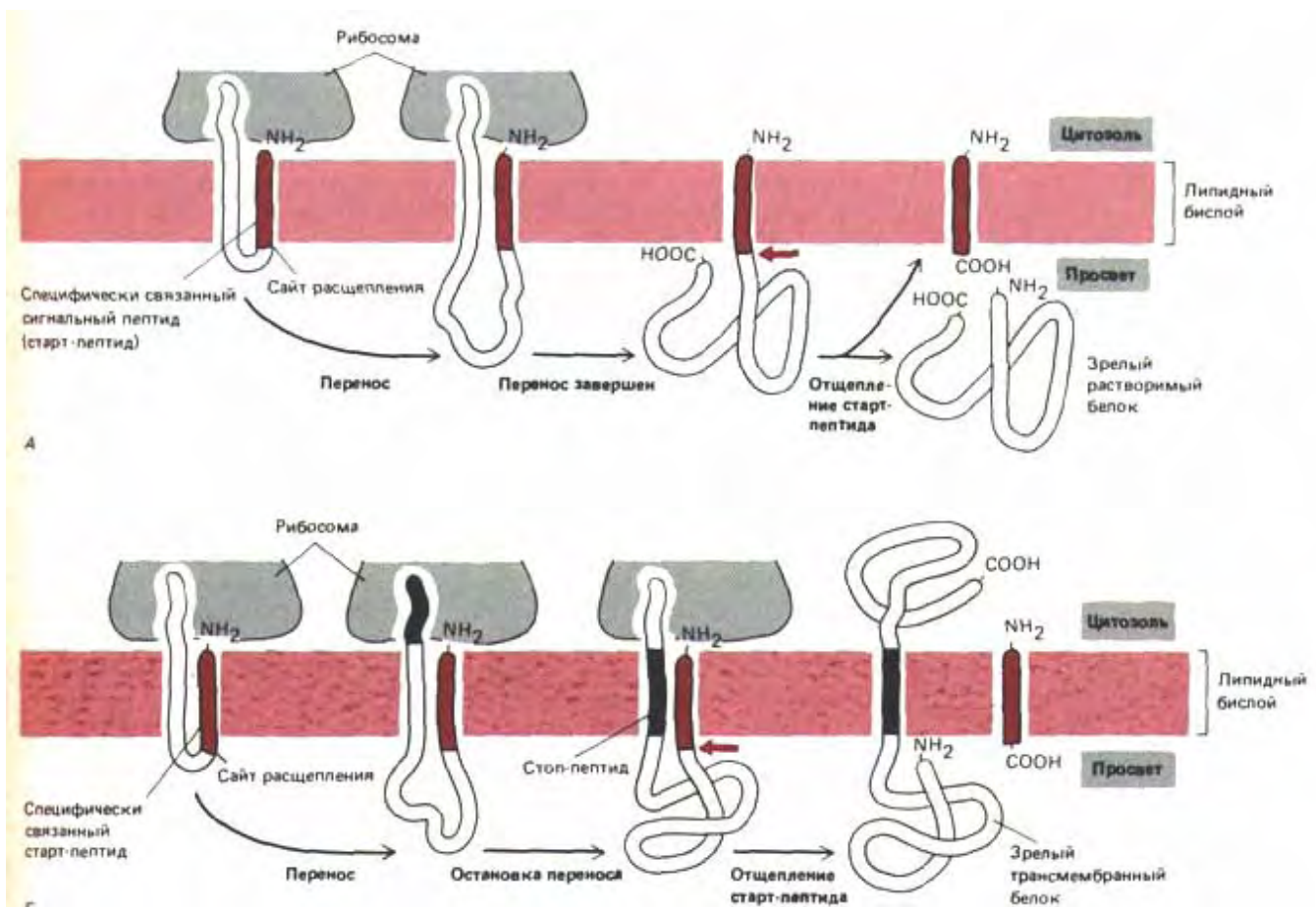
Рис. 8-45. Топология переноса белка через мембрану ЭР, проиллюстрированная для двух простых случаев. Считается, что промежуточный продукт переноса содержит петлю полипептидной цепи, в которой сигнальный пептид (называемый также сигналом начала переноса) формирует половину вертикального участка петли, а вторая половина в каждый данный момент образована переносимым участком полипептида. В случае, когда имеется только старт-пептид, а стоп-пептид отсутствует, полипептид переносится через мембрану целиком, и после отрезания стартового пептида в просвет (полость) ЭР высвобождается зрелый растворимый белок (А). Если имеется один старт-пептид и один стоп-пептид, перенос прекращается, когда стоп-пептид достигнет вертикального участка петли, в то время как синтез белка с цитозольной стороны мембраны продолжается; после отрезания сигнала начала переноса зрелый белок остается в мембране, он пронизывает липидный бислой ЭР, и с каждой стороны мембраны выступает по домену (В).
