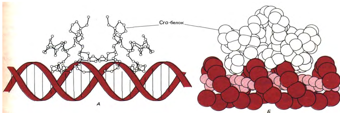
Рис. 9-12. Схема связывания сго-белка бактериофага лямбда с ДНК. Белок представляет собой симметричный гомодимер, который связывается с симметричной последовательностью ДНК, представленной на рис. 9-11. Способ связывания с ДНК определен путем анализа молекулярных моделей. А. Проволочная модель молекулы белка, совмещенная со схематическим изображением двойной спирали ДНК. Б.
