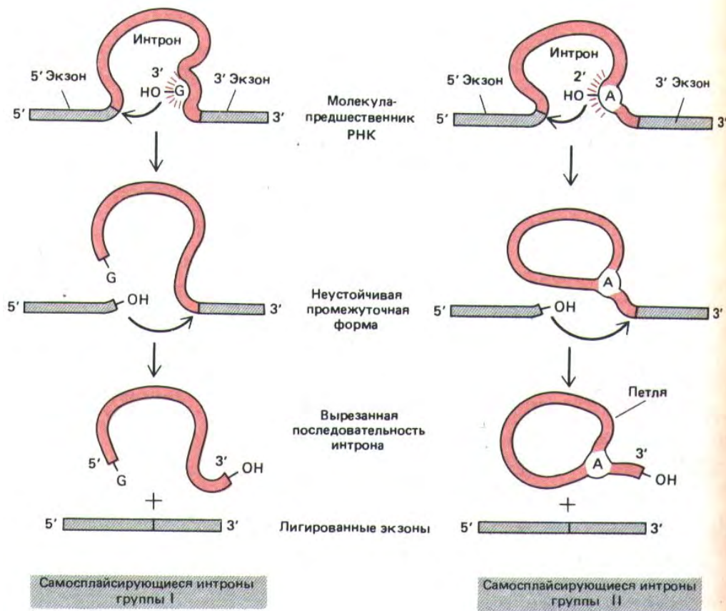
Рис. 9-87. Два известных класса самосплайсирующихся интронов. У интронов группы I для инициации сплайсинга с определенным сайтом связывается свободный G-нуклеотид (см. рис. 3-19), а у интронов группы II используется особым образом активированный A-нуклеотид. Эти две группы интронов изображены таким образом, чтобы были видны их общие свойства. В обоих случаях ускорение реакции определяется белками, но в катализе участвует и РНК, входящая в состав интрона. Механизм, используемый интронами группы II, приводит к образованию лассо-подобных структур и напоминает реакцию, катализируемую сплайсосомой (ср. рис. 9-82). (По Т.К. Cech, Cell 44: 207-210, 1986.)
