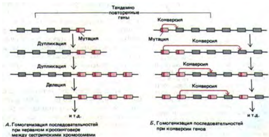
Рис. 10-64. Два типа событий, позволяющих сохранить последовательности ДНК в тандемном расположении и очень похожими друг на друга. А. Постоянное увеличение и уменьшение числа копий гена в тандеме при неравном кроссинговере (см. рис. 10-63) приводит к гомогенизации всех последовательностей генов, входящих в состав кластера. Б. При конверсии генов одна копия действует как матрица, которая передает либо все, либо часть последовательностей своей ДНК другой копии гена. У высших эукариот эти процессы, по-видимому, присущи генам, расположенным рядом друг с другом на хромосоме. У низших эукариот, например у грибов, конверсия генов у которых изучена гораздо лучше, этот процесс, как оказалось, не лимитирован лишь соседними генами.
