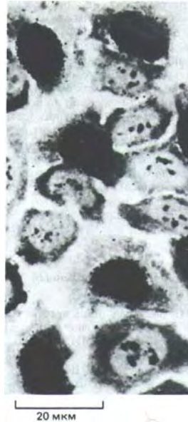
Рис. 13-2. Радиоавтограф, полученный после кратковременной инкубации клеток с ^3\text{H} -тимидином. Эта методика описана в разд. 4.5.2. Наличие зерен серебра в фотоэмульсии над ядрами (черные участки) свидетельствует о том, что клетки включали ^3\text{H} -тимидин в ДНК и, следовательно, в период экспозиции какое-то время находились в фазе S. (С любезного разрешения James Cleaver.)
