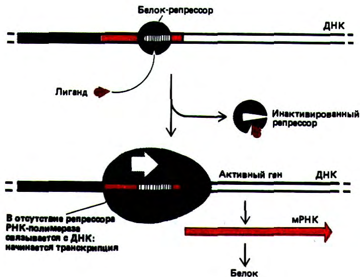
Рис. 10-11. Схема дерепрессии у бактерий. Небольшая специфическая молекула связывается с белком-репрессором, в результате чего происходит изменение его конформации и отделение от ДНК, при этом расположенные рядом гены могут начать транскрибироваться. В случае примера, описанного в тексте, аллолактоза связывается с белком-репрессором лактозного оперона, в результате чего синтезируется единственный транскрипт РНК, кодирующий три белка, которые участвуют в метаболизме лактозы ( \beta -галактозидаза, галакто-зидпермеаза и галактозидацетилаза). Поскольку три гена, кодирующие эти белки, расположены рядом друг с другом и их регуляция осуществляется строго координированно, кластер этих генов называют лактозным опероном.
