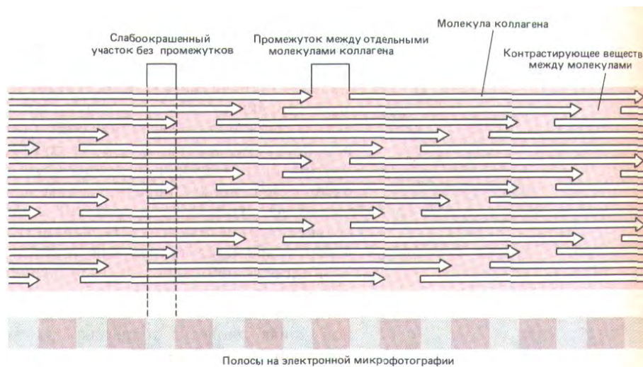
Рис. 14-36. Схема ступенчатого расположения молекул коллагена (они изображены в виде стрелок) в коллагеновой фибрилле. Молекулы в соседних рядах сдвинуты друг относительно друга на 67 нм, а промежутки между молекулами в продольном ряду составляют 35 нм. При такой величине этого промежутка продольное расположение молекул повторяется через каждые пять рядов, так что, например, молекулы в рядах 1 и 6 лежат точно друг против друга.
