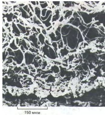
Рис. 14-43. Густая сеть эластических волокон в срезе соединительной ткани кожи (дермы) человека. Микрофотография, полученная с помощью сканирующего электронного микроскопа. Для того чтобы убрать collagen и гликоз-аминогликаны, ткань подвергали нагреву под давлением. (T. Tsuji, R. M. Lavker, A. M. Kligman. J. Microscop. 115: 165-173, 1978.)
