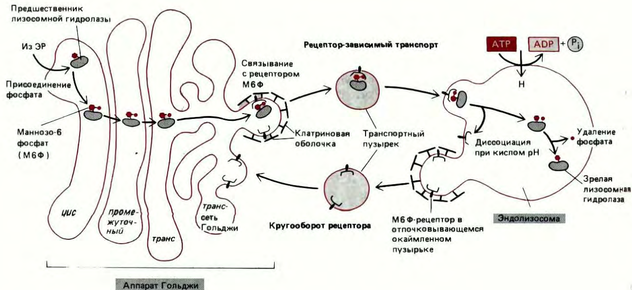
Рис. 8-72. Транспорт вновь образованных лизосомных гидролаз в лизосомы. В цис-аппарате Гольджи предшественники лизосомных гидролаз «метятся» при помощи маннозо-6-фосфатных групп, а в транс-сети Гольджи отделяются от других типов белков. Это отделение происходит потому, что отпочковывающиеся от транс-сети Гольджи клатриновые окаймленные пузырьки содержат рецепторы маннозо-6-фосфата, связывающие лизосомные гидролазы. Пузырьки утрачивают «кайму» и сливаются с эндолизосомами (см. рис. 8-71). При низком pH, который существует в эндолизосомах, гидролазы отщепляются от рецепторов. Рецепторы возвращаются в аппарат Гольджи для проведения повторных циклов транспорта. Вероятность возвращения гидролазы в аппарат Гольджи вместе с рецептором сильно снижается за счет удаления фосфата от маннозного остатка. Хотя существует два структурно различных маннозо-6-фосфат-рецепторных гликопротеина, сильно отличающихся по размерам, они имеют сходную аминокислотную последовательность и, вероятно, выполняют сходные функции.
