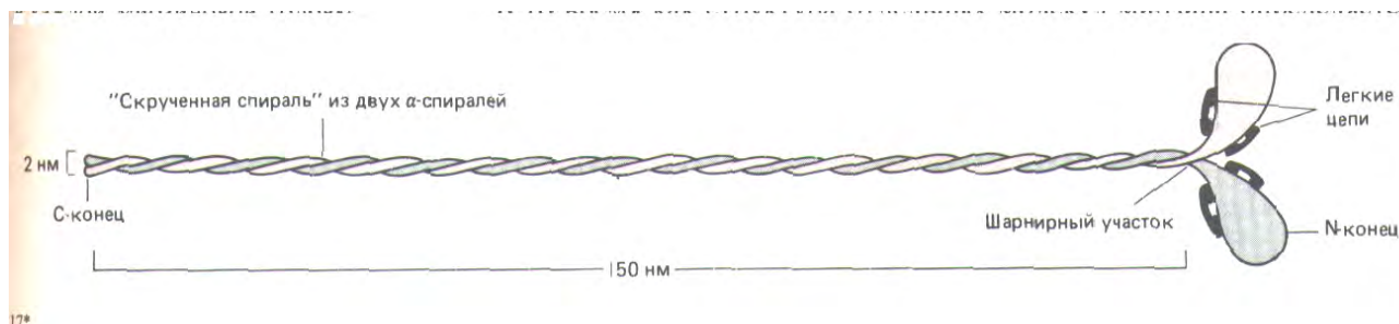
Рис. 11-9. Молекула миозина построена из двух тяжелых цепей (каждая длиной около 2000 аминокислотных остатков) и четырех легких цепей. Легкие цепи представлены молекулами двух типов (в одних около 190 аминокислотных остатков, в других около 170)-по одной молекуле каждого типа в каждой миозиновой головке.
