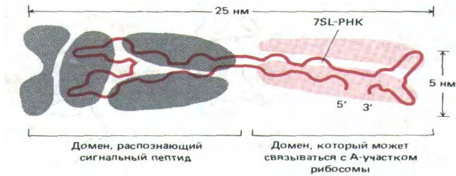
Рис. 8-42. Сильно упрощенная схема частицы, распознающей сигнал (SRP). Она представляет собой вытянутый комплекс, состоящий из шести полипептидных цепей (закрашенные участки) и одной молекулы 7SL-PHK. Один конец этой частицы связывается с рибосомой, а другой — с сигнальным пептидом вновь синтезированной полипептидной цепи. Было сделано предположение, что часть 7SL-PHK может сворачиваться в тРНК-подобную структуру, которая конкурирует в А-участке рибосомы с поступающими аминоксил-тРНК, вызывая, таким образом, паузу в трансляции. (По V. Stegel и P. Walter, Nature 320: W-84, 1986.)
