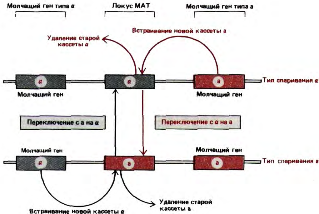
Рис. 10-30. Кассетная модель переключения типа спаривания у дрожжей. Кассетное переключение происходит в ходе процесса конверсии гена, запускаемого, когда нуклеаза НО делает двухцепочечный разрез в определенной последовательности ДНК локуса МАТ. ДНК вблизи разреза затем удаляется и заменяется копией молчащей кассеты, определяющей противоположный тип спаривания.
