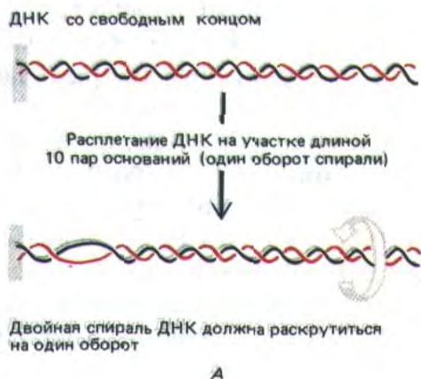
Рис. 10-41. Напряжение, возникающее при суперспирализации ДНК, приводит к суперскручиванию молекулы. А. У молекулы ДНК с одним свободным концом (либо разрывом в одной из цепей, который служит шарниром) двойная цепь раскручивается на один виток на каждые 10 неспаренных нуклеотидных пар. Б. Если вращению что-либо препятствует, супервитки вводятся в ДНК путем раскручивания спирали в другом месте. В результате на каждые 10 неспаренных нуклеотидных пар возникает один супервиток. На этом рисунке изображена положительная суперспираль (см. рис. 10-42).
