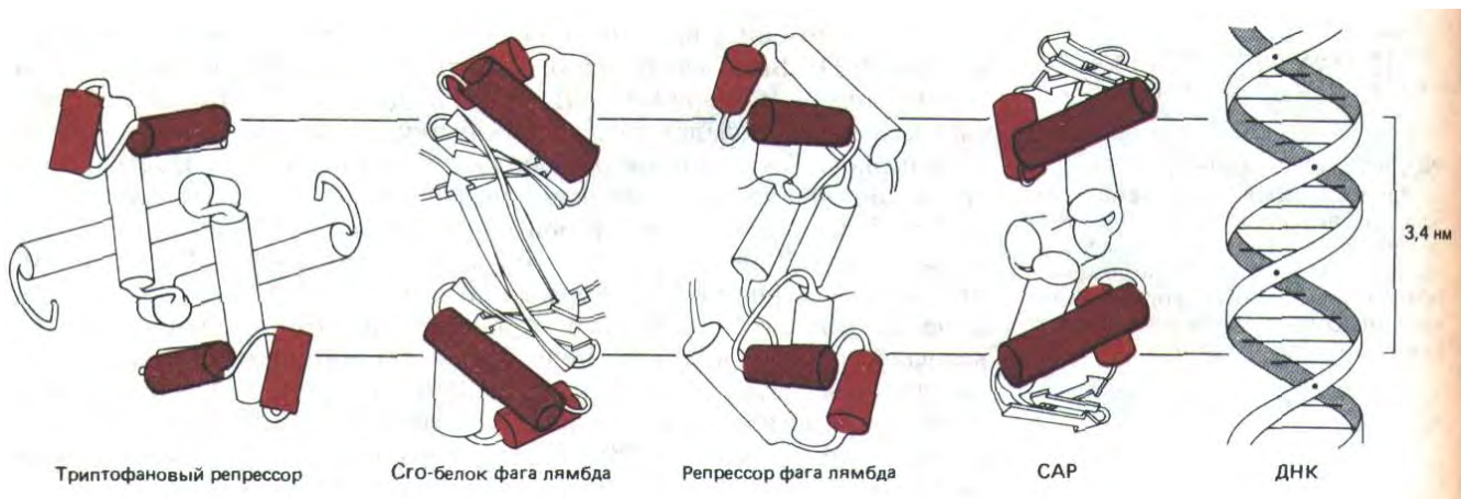
Рис. 9-13. Семейство димерных ДНК-связывающих белков. Эти регуляторные белки работают в бактериальных системах: репрессор лямбда и сго-белок контролируют экспрессию генов бактериофага лямбда, а белок активатор катаболизма (CAP) регулирует экспрессию ряда генов E. coli , которые могут включаться лишь в отсутствие глюкозы. В каждом случае рентге-ноструктурный анализ выявил наличие двух копий узнающей спирали (коричневый цилиндр), разделенных одним витком спирали ДНК (3,4 нм).
