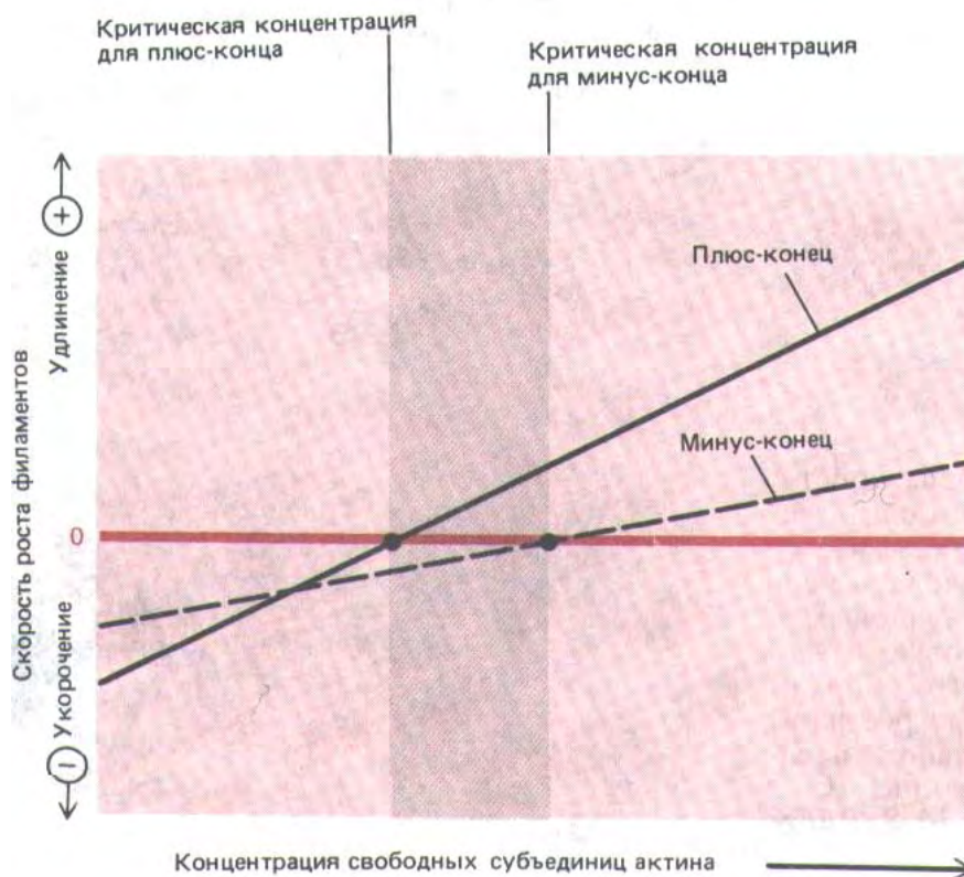
Рис. 11-41. Скорость роста активных филаментов на разных концах при различных концентрациях мономеров актина. График показывает, что два конца растут с разными скоростями и критические концентрации для них различны. Поэтому существует некоторый диапазон концентраций свободного актина (темная полоса), при которых плюс-конец активного филамента полимеризуется, а минус-конец деполимеризуется. Когда in vitro свободный актин находится в равновесии с активными филаментами, в целом роста не происходит, так как скорости отделения молекул от минус-конца и присоединения их к плюс-концу равны. При такой концентрации свободных активных субъединиц (промежуточной между критическими концентрациями для двух концов-показано цветной стрелкой) длина филаментов не изменяется, но молекулы актина в них все время движутся от одного конца полимера к другому. Этот процесс называют тредмил-лингом (см. схему 11-1).
