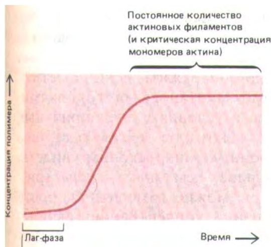
Рис. 11-39. Кинетика полимеризации актина in vitro . Полимеризацию инициируют повышением ионной силы в растворе актина, и она обычно начинается после некоторой выдержки (лаг-фазы).
