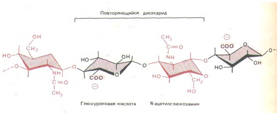
Рис. 14-25. Повторяющаяся дисахаридная последовательность гиалуроновой кислоты - относительно простого гликозаминогликана, состоящего из одной очень длинной цепи, в которой может быть до нескольких тысяч сахарных остатков. Обратите внимание на отсутствие сульфатных групп.
