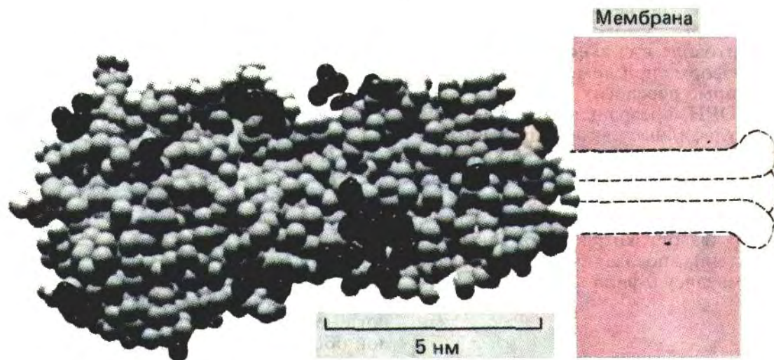
Рис. 8-51. Трехмерная структура мембранного гликопротеина-гемагглютинина вируса гриппа, показывающая расположение в нем ковалентно присоединенных олигосахаридов (выделенные темными атомы). Гликопротеины либо встраиваются в клеточные мембраны, либо выводятся из клеток при секреции; они могут содержать от 1 до 85% углеводов по весу. Некоторые богатые углеводами гликопротеины содержат десятки или даже сотни присоединенных олигосахаридных цепей на молекулу. Пронизывающие мембрану участки этого белка вирусной оболочки, состоящие из трех идентичных полипептидных цепей, могут служить основанием представленной здесь структуры. Они не изображены на рисунке, т. к. этот участок белка отрезается при приготовлении образца для рентгено-структурного анализа. (Фотографию любезно предоставил Richard J. Feldmann.)
