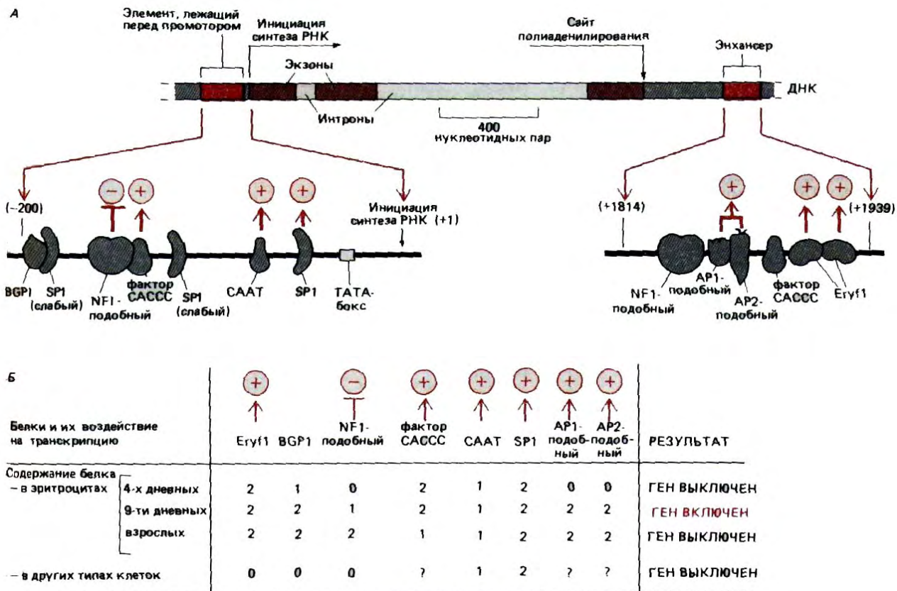
Рис. 10-23. Известные белки-регуляторы, контролирующие экспрессию гена \beta -глобина курицы в ходе нормального развития эритроцита. Здесь суммированы данные экспериментов, описанных на рис. 10-20 и 10-21; аналогичных опытов, проведенных с мутантными элементами, расположенными перед промотором, а также результаты анализа другого типа. А. Связывающие участки белков-регуляторов и их действие. Следует отметить, что энхансер у этого гена расположен за кодирующей последовательностью. Белки, не отмеченные + (активация) или — (подавление), по-видимому, не оказывают существенного влияния на транскрипцию, поскольку мутация их сайта связывания не сказывается на уровне транскрипции (см. рис. 10-21). Б. Относительные количества регуляторных белков на разных стадиях развития. Числами 0, 1 и 2 обозначено отсутствие, промежуточный и высокий уровень транскрипции соответственно, по нелинейной шкале. Имеющиеся в настоящее время данные не дают точного объяснения, почему ген включается между 4 и 9 днями развития. (С любезного разрешения Gary Felsenfeld.)
