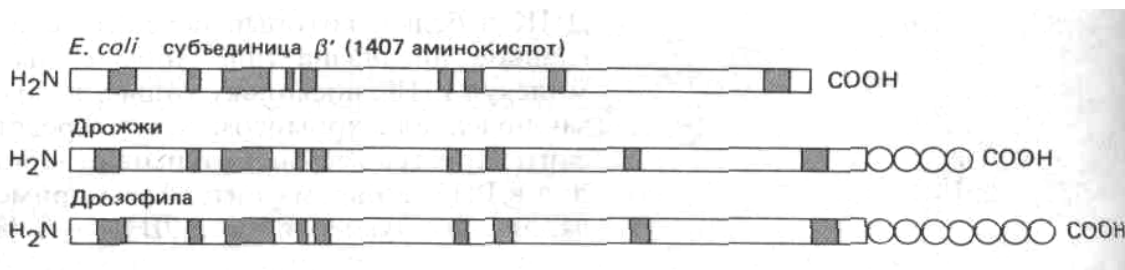
Рис. 9-64. Сходство аминокислотной последовательности бактериальных и эукариотических РНК-полимераз дает основание предположить, что эти ферменты имеют общее эволюционное происхождение. Полагают, что с ДНК связываются самые большие субъединицы РНК-полимераз из клеток E. coli , дрожжей и дрозофилы (они сравниваются на рисунке). Закрашенные участки последовательности гомологичны более, чем на 70% у дрожжей и дрозофилы и более, чем на 40% - у дрозофилы и E. coli . Показано, что на карбоксильном конце эукариотических субъединиц имеется уникальная последовательность Ser-Pro-Ser-Tyr-Ser-Pro-Thr, функция которой неизвестна: у дрожжей она повторяется 26 раз, а у дрозофилы - более 40 раз (обозначено кружками), (По A. Z. Green-leaf et al., In: RNA Polymerase and the Regulation of Transcription [W.S. Reznikoff et al., eds.] pp. 459-464. New York: Elsevier, 1987.)
