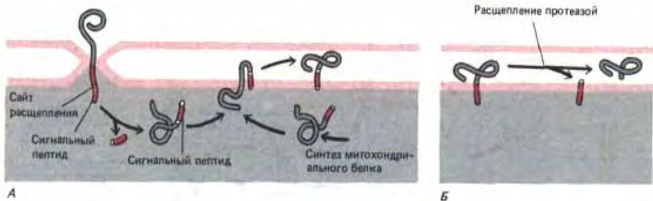
Рис. 8-30. Импорт белков из цитозоля в межмембранное пространство митохондрий или внутреннюю мембрану требует многих сигналов. Вначале белок переносится в пространство матрикса, как это показано на рис. 8-29. Однако при отрезании сигнального пептида, использованного для первичного переноса, обнажается смежный гидрофобный сигнальный пептид на новом N-конце. Этот сигнал вызывает встраивание белка во внутреннюю мембрану таким же образом, каким в нее встраиваются белки, кодируемые митохондриальным геномом (А.) Этот механизм предположительно сходен с тем, который бактериальные предки митохондрий использовали для встраивания белков в плазматическую мембрану, и, как полагают, напоминают механизм встраивания белков в ЭР. Для транспорта белков в межмембранное пространство требуется еще третья стадия, на которой протеаза с активным центром, обращенным в трансмембранное пространство, отрезает белок от его трансмембранного сигнального пептида, находящегося во внутренней мембране (Б). Путь, изображенный на рис. (А), может быть использован и для переноса белков из цитозоля во внутреннюю мембрану, который тоже требует гидрофобного пептида.
