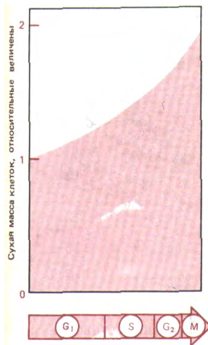
Рис. 13-7. График увеличения массы клеток за время клеточного цикла. Большая часть клеточных компонентов синтезируется более или менее равномерно на протяжении всей интерфазы, причем скорость их образования обычно возрастает по мере того, как размеры клетки и ее биосинтетическая активность увеличиваются (с коротким перерывом в фазе М). Чтобы в пролиферирующей популяции средняя величина клетки оставалась постоянной, количество каждого компонента за время цикла должно в точности удваиваться. метод состоит в том, что используют изменения цитоскелета в М-фазе, приводящие к «округлению» клеток. Округлившись в М-фазе клетки так слабо прикрепляются к дну культуральной чашки, что их можно отделить легким встряхиванием (рис. 13-6). Митотические клетки, отобранные таким способом, составляют синхронную популяцию, в которой почти сразу же наступает фаза G_1 клеточного цикла. Применяют и другой метод: поскольку клетки по мере прохождения цикла увеличиваются в размерах, можно использовать центрифугирование, чтобы выделить субпопуляции клеток, находящихся на разных стадиях цикла.
