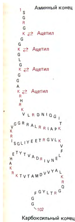
Рис. 9-21. Аминокислотная последовательность гистона Н4-одного из нуклеосомных гистонов. Аминокислоты обозначены однобуквенными сокращениями, положительно заряженные аминокислоты выделены цветом. Как и в случае других нуклеосомных гистонов, протяженная аминоконцевая последовательность молекулы обратимо модифицируется в клетке путем ацетилирования отдельных остатков лизина. Приведенная последовательность соответствует гистону Н4 быка. У гороха этот гистон имеет почти такую же аминокислотную последовательность, за исключением того, что в нем один остаток валина замещен на изолейцин, а один остаток лизина - на аргинин.
