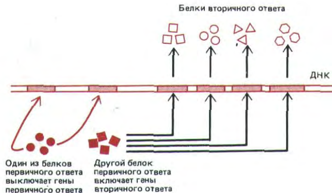
Рис. 12-11. Схема раннего первичного (А) и задержанного вторичного (Б) ответа клеток дрозофилы на экдизон. Некоторые из белков, синтезируемых при первичном ответе, включают гены, ответственные за вторичный ответ, а другие выключают гены, участвовавшие в первичном ответе. На самом деле в обоих ответах участвует больше генов, чем показано на схеме.
