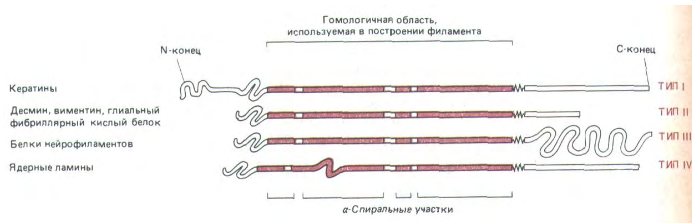
Рис. 11-74. У всех белков промежуточных филаментов имеется гомологичная центральная область (около 310 аминокислотных остатков), формирующая протяженную \alpha -спираль с тремя короткими участками иной структуры. N-концевой и С-концевой домены не состоят из \alpha -спирали и сильно варьируют по размерам и последовательности аминокислот у белков разных промежуточных филаментов.
