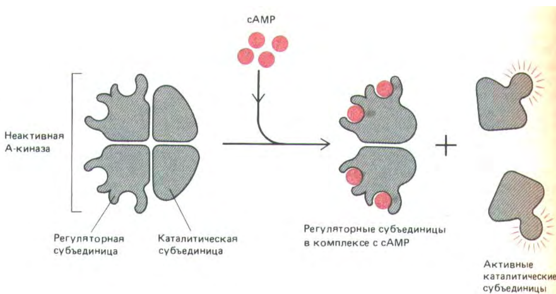
Рис. 12-27. Активация cAMP-зависимой протеинкиназы (А-киназы). Присоединение cAMP к регуляторным субъединицам фермента вызывает изменение их конформации, приводящее к отделению этих субъединиц от комплекса. Освобождаемые при этом каталитические субъединицы активируются. Каждая регуляторная субъединица имеет два участка для связывания cAMP, и освобождение каталитических субъединиц представляет собой кооперативный процесс, требующий присоединения более чем двух молекул cAMP на тетрамер. Это делает реакцию киназы на изменение концентрации cAMP значительно более резкой (см. разд. 12.4.8). Во многих клетках имеются А-киназы двух типов - одинаковыми каталитическими субъединицами, но разными регуляторными.
