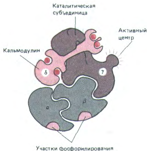
Рис. 12-31. Сильно схематизированное изображение четырех субъединиц киназы фосфоорилазы из мышц млекопитающих. Каталитической активностью обладает \gamma -субъединица; \alpha - и \beta -субъединицы участвуют в регуляции этой активности циклическим АМР, а \delta -субъединица (кальмодулин) - в ее регуляции ионами \text{Ca}^{2+} . В действительности полный ферментный комплекс содержит по четыре копии каждой субъединицы.
