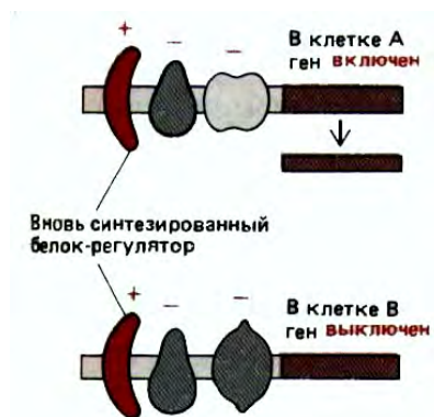
Рис. 10-8. Воздействие вновь синтезированных белков-регуляторов на клетку. Подобное воздействие зависит от того, какие белки-регуляторы уже имеются в клетке и, следовательно, от ее предыстории. На схеме один и тот же ген изображен в клетках А и В. Изначально этот ген в обеих клетках выключен. Однако в клетке А продуцируется белок, изображенный крайним слева и отсутствующий в клетке В. Для простоты принимается, что каждый белок-регулятор либо положительно, либо отрицательно воздействует на транскрипцию, которая определяется их совместным воздействием. В действительности же общее воздействие не обязательно осуществляется по принципу аддитивности. Например, в некоторых случаях два белка-регулятора при связывании с ДНК взаимодействуют друг с другом, причем происходит изменение активности каждого из них.
