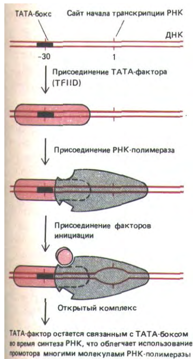
Рис. 9-69. Минимальные условия для узнавания промотора молекулой эукариотической РНК-полимеразы II. Чтобы промотор был узнан полимеразой, необходимо, чтобы фактор связывания с ТАТА-боксом (TFIID) образовал стабильный транскрипционный комплекс. Консенсусная последовательность ТАТА-бокса следующая: T 82 A 9 T 93 A 85 (А или Т) 83 , числа указывают на вероятность (в процентах) присутствия указанного нуклеотида. См. также рис. 10-27. (По J.2. Workman and R.G. Roeder, Cell 51: 613-622, 1987.)
