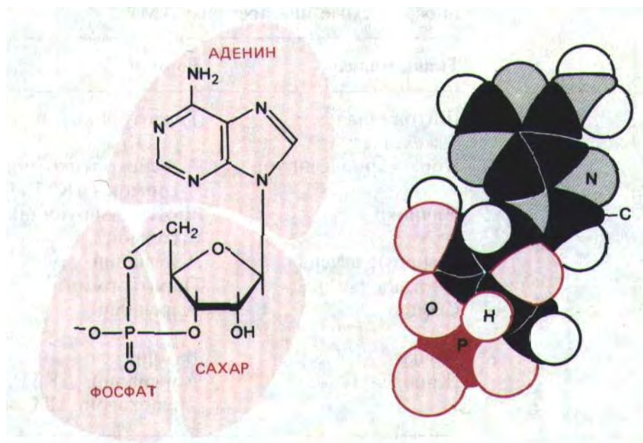
Рис. 12-14. Структурная формула и объемная модель циклического AMP (C, H, N, O и P-атомы углерода, водорода, азота, кислорода и фосфора соответственно).
