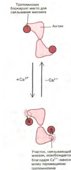
Рис. 11-19. Актиновый филамент в поперечном разрезе (схема): показано, каким образом в отсутствие \text{Ca}^{2+} тропомиозин может блокировать взаимодействие миозиновых головок с актином.
