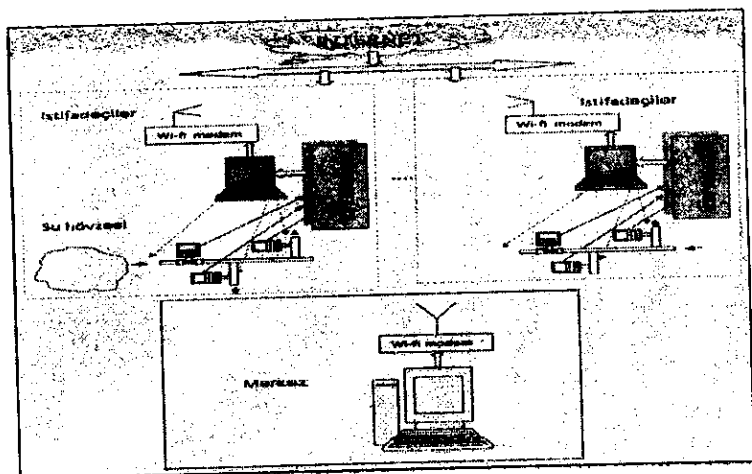
Şəkil 10.15. Su təchizatı sisteminin lokal şəbəkələrinin birliyin korporativ informasiya şəbəkəsi ilə əlaqə sxemi
