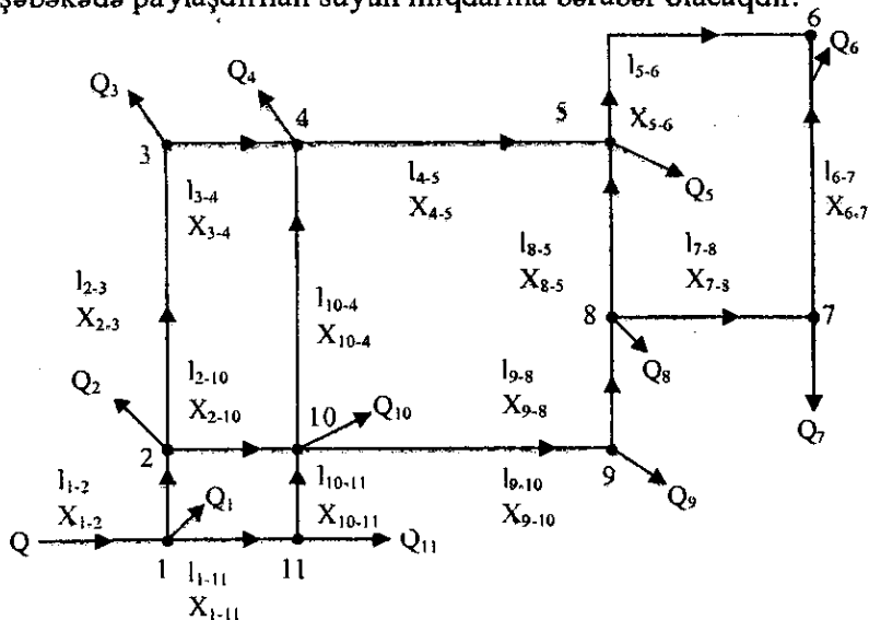
Şəkil 10.8. Şəbəkədə məntəqələr üzrə suyun paylanması
