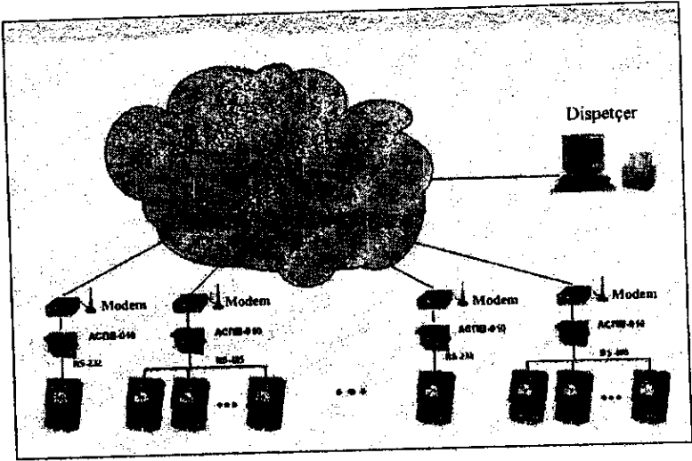
Şəkil 10.10. Sayğacların göstəricilərinin İİM-nə simsiz rabitə sistemi ilə göndərilməsinin GSM variantı
