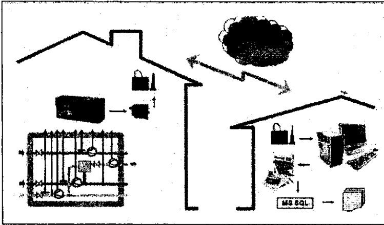
Şəkil 10.12. İİS-nin GSM mühitində texniki vasitələr kompleksinin əlaqə sxemi
