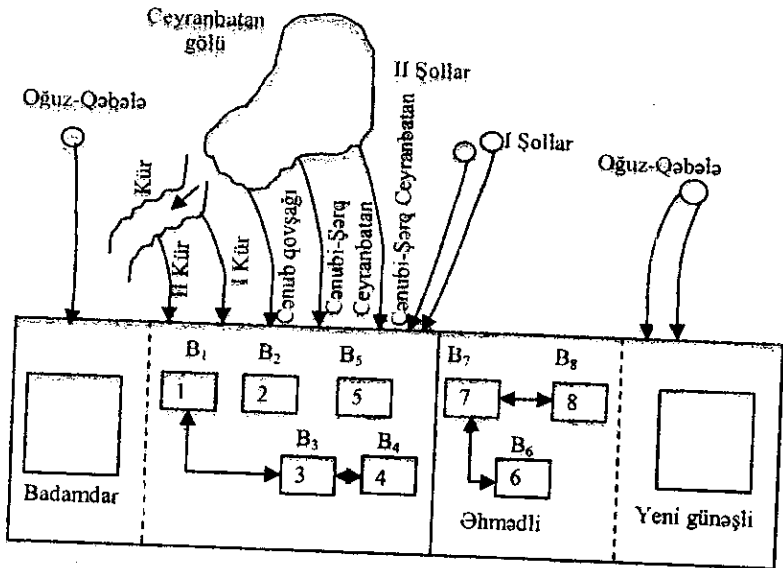
Şəkil 10.13. Su təchizatının sadələşdirilmiş struktur sxemi
