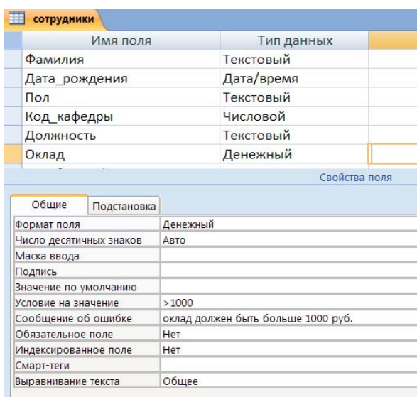
Рис. 5.41. Задание ограничений целостности при описании полей таблицы
