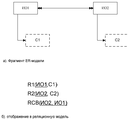
Рис. 3.3. Отображение связи М:М
