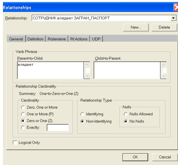
Рис. 4.73. Описание связи «СОТРУДНИК - ЗАГРАНПАСПОРТ»
