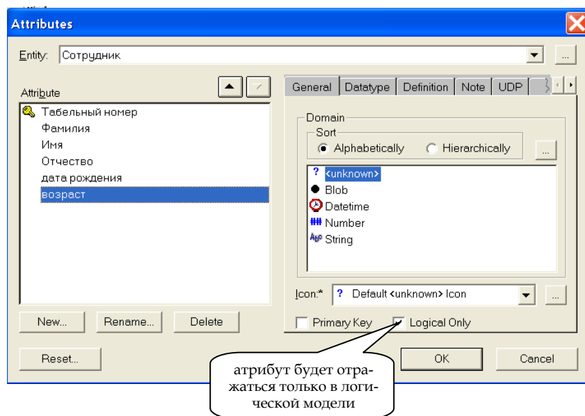
Рис. 4.19. Использование признака Logical Only
