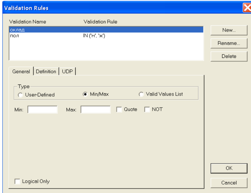
Рис. 4.66. Задание диапазона значений атрибута
