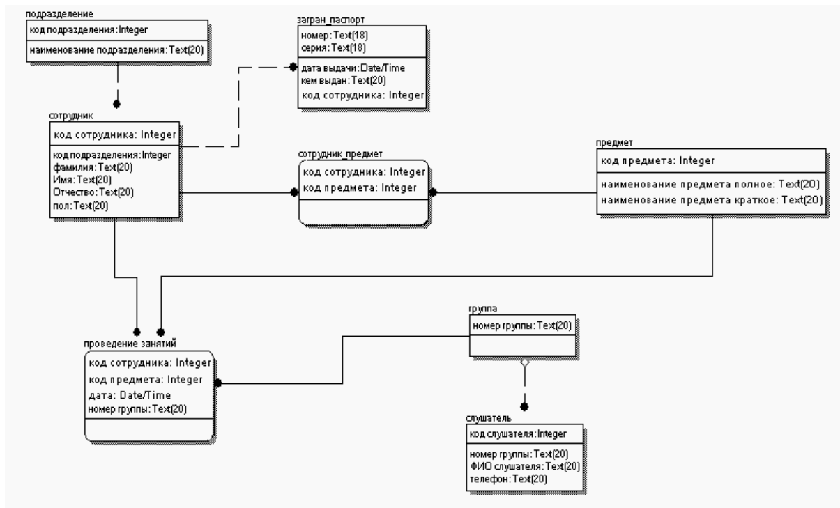
Рис. 4.82. Физическая модель в нотации IDEF1X1X
