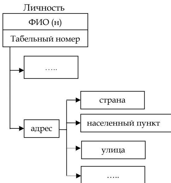
Рис. 2.10. Пример изображения составного свойства
