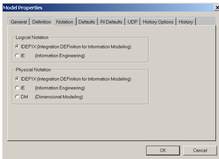
Рис. 4.9. Выбор нотации
