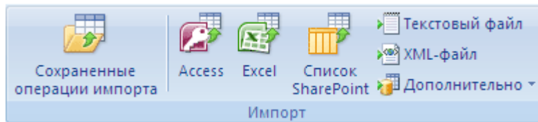
Рис. 5.31. Импорт данных
