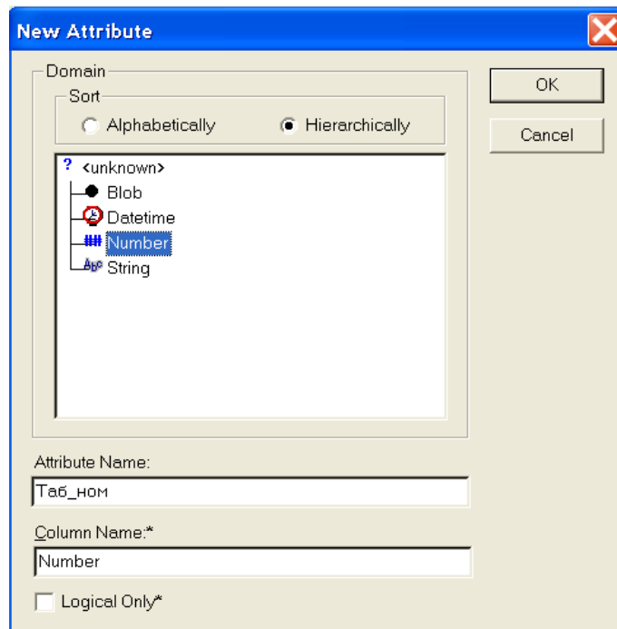
Рис. 4.17. Описание атрибута
