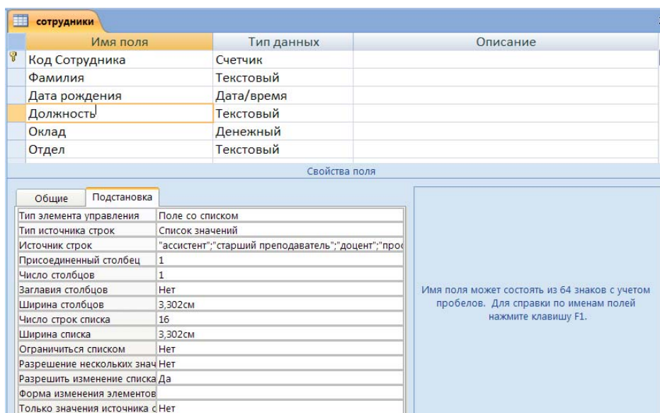
Рис. 5.15. Свойства подстановки
