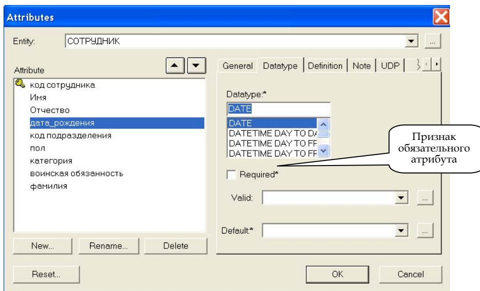
Рис. 4.61. Окно описания атрибутов. Вкладка Datatype
