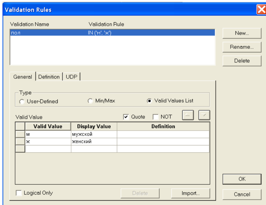
Рис. 4.64. Задание списка допустимых значений атрибутов
