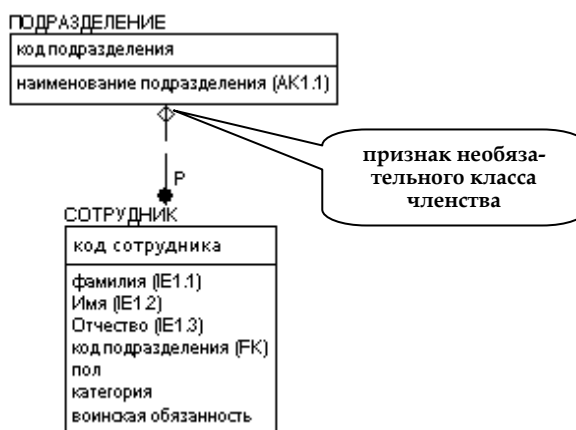
Рис. 4.44. Пример неидентифицирующей связи с необязательным классом членства
