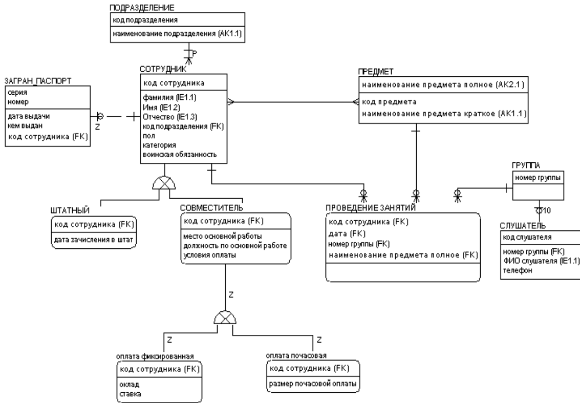
Рис. 4.55. Вид модели в нотации IE
