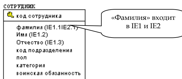
Рис. 4.28. Сущность «Сотрудник». Задан первичный ключ и два инверсных входа
