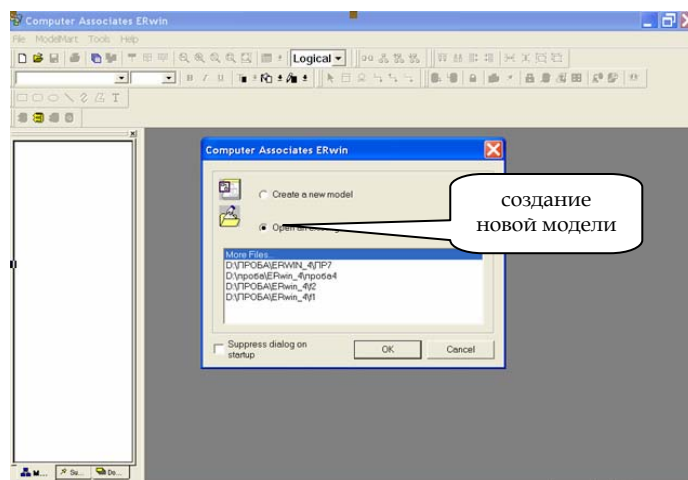
Рис. 4.1. Начальный экран
