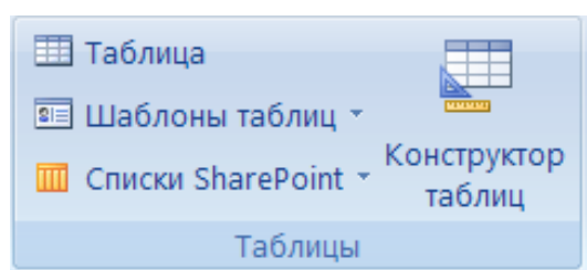
Рис. 5.8. Блок Таблицы
