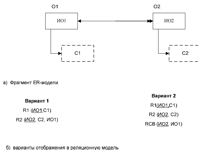
Рис. 3.4. Отображение связи 1:М
