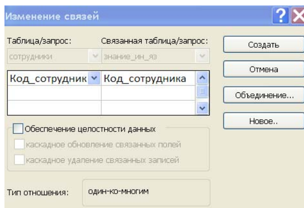
Рис. 5.39. Задание связи и ограничений целостности по связи
