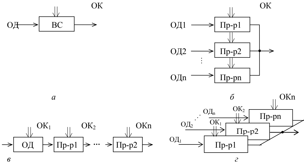
Рис. 1.1.9. Архитектура ВС: а– ОКОД (SISD) – архитектура; б– ОКМД (SIMD) – архитектура; в– МКОД (MISD) – архитектура; г– МКМД (MIMD) – архитектура
