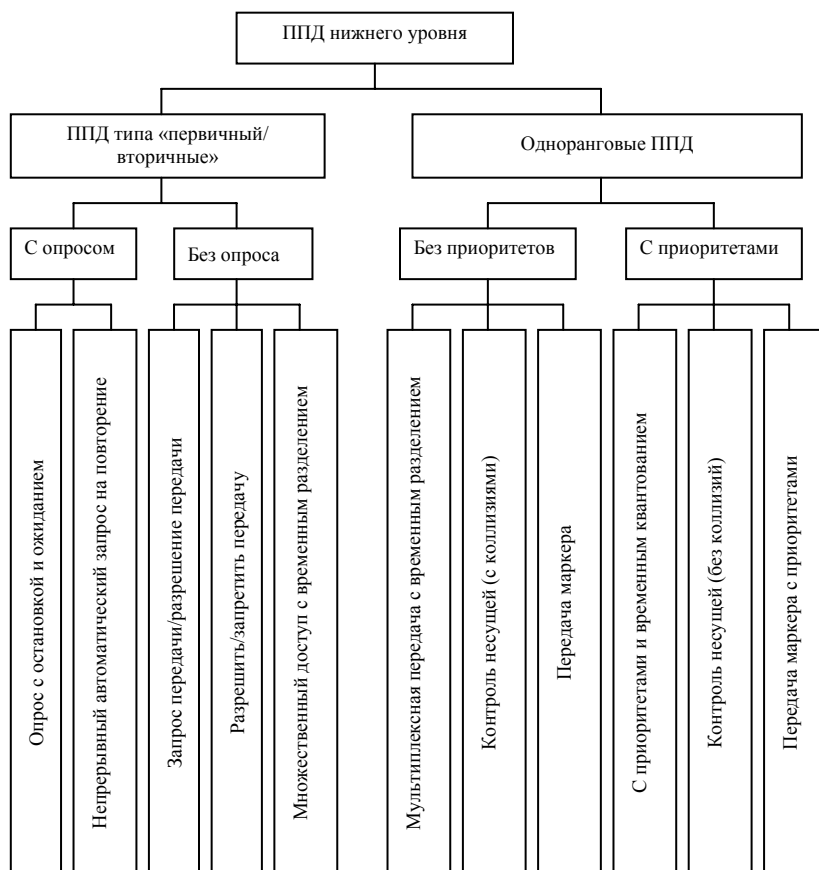
Рис. 29. Классификация ППД нижнего уровня
