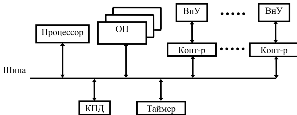
Рис. 4. Структурная схема ПК
