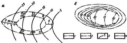
Рис. 16. Схема построения карты эффективных нефтенасыщенных мощностей а - карта эффективных мощностей с внешним и внутренним контурами нефтеносности; б - карта эффективных нефтенасыщенных мощностей; 1 и 2 - внешний и внутренний контуры нефтеносности; 3 - изопахиты эффективных мощностей; 4 - изопахиты нефтенасыщенных мощностей
