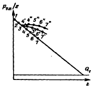
Рис.31. График динамики разработки газовой залежи: линии: 1-7 - газовый режим 1'-2'-3'-4'-5'-6' - газо-упруго-водонапорный режим 1''-2''-3''-4''-5''-6''-7'' - газоводонапорный режим
