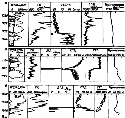
Рис 82. Примеры выделения работающей мощности пластов:
