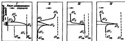
Рис.81. Типовые диаграммы термокондуктивного дебитомера против интервала притока:
