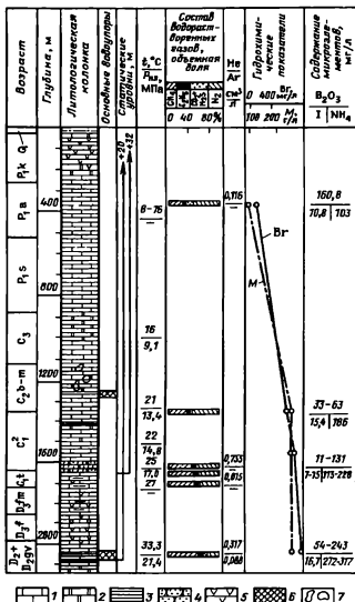
Рис. 63. Гидрогеологический разрез Ярино-Каменоложского месторождения (по И.Н. Шестову):
