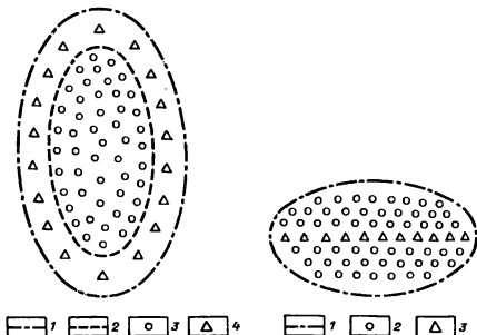
Рис. 73. Система разработки нефтяных залежей с приконтурным заводнением: 1 и 2 - внешний и внутренний контуры нефтеносности; скважины: 3 - добывающие, 4 - нагнетательные
