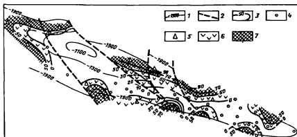
Рис.64. Карта распределения нагнетаемой воды в заводненном объеме верхнемеловой залежи месторождения Карабулак-Ачалуй по состоянию на 01.01.1964 г. (по А.М. Никанорову):
