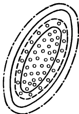
Рис.71. Система разработки нефтяных залежей с использованием естественного напора пластовых вод: 1 и 2 - контуры нефтеносности: внешний и внутренний; 3 - изогибсы пласта; 4 - добывающие скважины
