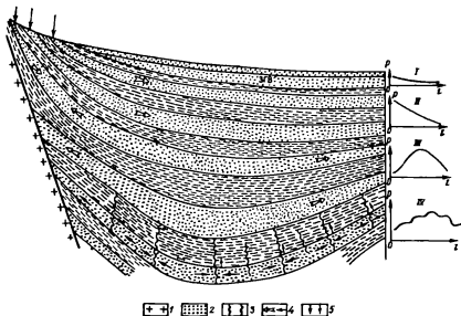
Рис.53. Схема гидродинамической зональности в бассейнах пластовых вод: 1 - кристаллический массив, 2 - водонапорная система, 3 - трещиноватость, 4 - направление движения, 5 - инфильтрация метеогенных вод. Зоны: I - распространения грунтовых геогидродинамических систем, II - распространения инфильтрационных природных еодонапорных систем, III - распространения элизионных природных водонапорных геостатических систем, IV - возможного распространения термодегидратационных природных водонапорных систем; ЗГВ - зеркало грунтовых вод
