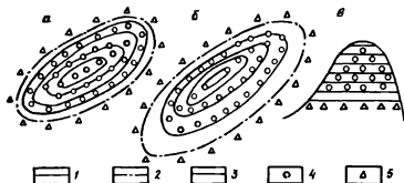
Рис.72 Система разработки нефтяной залежи с применением законтурного заводнения: а - симметричной сводовой, б - асимметричной сводовой в - литологически экранированной; 1 - изогипсы пласта, 2 - внешний контур нефтеносности, 3 - линия литологического ограничения скважины, 4 - добывающие, 5 - нагнетательные
