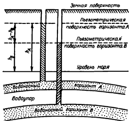
Рис. 65. Схема соотношений водоносных горизонтов с различными напорами для оценки условий хранения газов и жидкостей и захоронения промышленных стоков в водоносных пластах (по П. Уизерстуну и др.)
