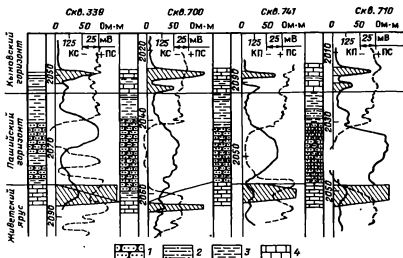
Рис. 8. Детальная (зональная) корреляция геолого-геофизических разрезов нижне-франкских отложений Шаповской площади (по В.А. Долицкому);
