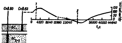
Рис. 62. Выявление гидродинамической связи пластов в разрезе месторождения (кривая изменения устьевое давления в скв.62 пласта БС 1 от пуска и остановки скв.80 пласта БС 2+3 Усть-Балыкского месторождения), по Ю.П. Гаттенбергеру, В.П. Дьяконову: 1 - пуск в эксплуатацию скв.80, 2 - остановка скв.80
