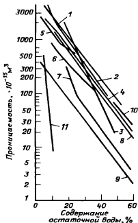
Рис. 24. Зависимость содержания остаточной воды от проницаемости для различных нефтегазоносных пород (по А.А. Ханину):
