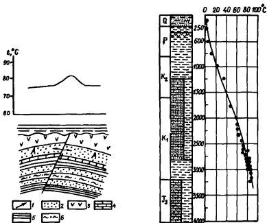
Рис.46. Схема образования гидрогеотермической аномалии в пласте А: 1 - направление движения вод по разлому; 2 - водоносный пласт; 3 - соленосная толща; 4 - пласт известняка; 5 - глинистый пласт; 6 - пласт алевролитов
