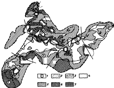
Рис.21. Схематическая карта изменения K_{неод} по свабжинам D_1 Серафимовского месторождения. 1 - номер расчетного участка; 2 - зоны отсутствия коллекторов; 3 - первоначальные внутренний и внешний контуры нефтеносности; 4 - K_{неод} < 1 ; 5 - K_{неод} = 1 \div 5 ; 6 - K_{неод} = 5 \div 10 ; 7 - K_{неод} > 10
