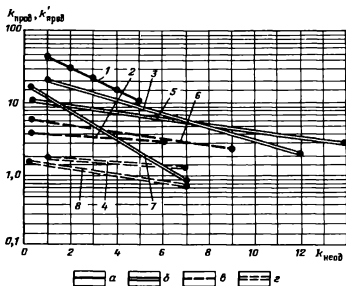
Рис.22. Зависимость коэффициентов продуктивности K_{\text{прод}} и удельной продуктивности K'_{\text{прод}} от K_{\text{неод}} для первой и второй групп объектов:
