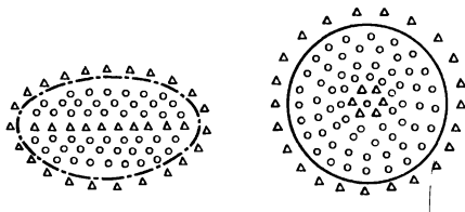
Рис. 75. Система разработки нефтяных залежей при сочетании осевого и законтурного заводнения:
