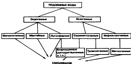
Рис. 54. Схема генетической классификации вод (по А.А. Карцеву)
