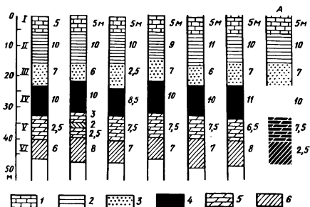
Рис. 11. Схема построения нормального (типового) разреза (А) продуктивной толщи 1 - известняки; 2 - аргиллиты; 3 - песчаники; 4 - нефть; 5 - доломиты; 6 - мергели
