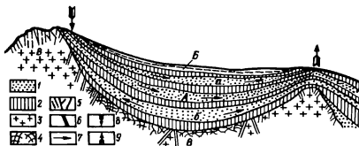
Рис. 49. Схема гидрогеологического бассейна. Породы: 1 - коллекторы; 2 - водоупоры; 3 - магматические; 4 - метаморфические; 5 - система трещин в магматических породах; 6 - тектонические нарушения; 7 - направление движения пластовых вод; 8, 9 - области соответственно питания и разгрузки вод. А - бассейн пластовых вод; Б - суббассейн грунтовых вод; В - бассейн трещинных и жильно-трещинных вод; природные водонапорные системы: а - инфильтрационные, б - элизионные
