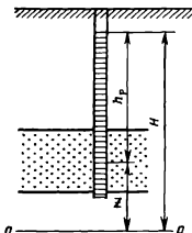
Рис.43. Графическое изображение пьезометрического напора
