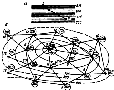
Рис. 14. Схема построения структурной карты способом треугольников: а - высотная арфа; б - структурная карта (цифрами в кругах показаны отметки пласта)
