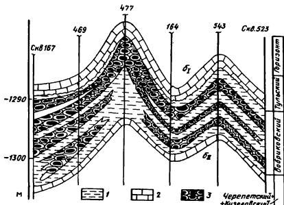
Рис. 13. Схема построения геологического разреза по линии профиля I-I 1 - глины; 2 - известняки; 3 - нефтенасыщенный песчаник
