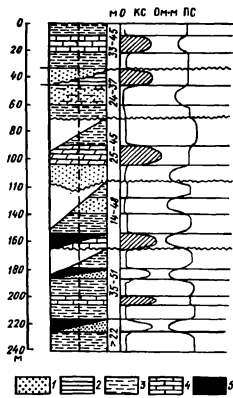
Рис. 12. Схема построения средненормального геолого-геофизического разреза месторождения (по В.А. Долицкому): 1 - пески; 2 - аргиллиты; 3 - глина; 4 - известняки; 5 - нефть
