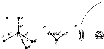
Рис.40 Модель молекулы воды: а - схема тетраэдрического характера водородной связи в воде, б - угол связи в молекуле воды; в - образование диполями воды ассоциированных молекул (дигидроля, тригидроля)
