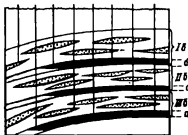
Рис. 69. Схема разработки многопластового нефтяного месторождения по системе снизу вверх
