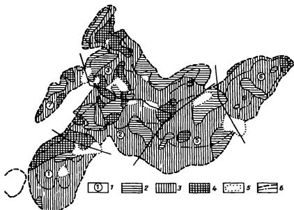
Рис. 19. Схема изменения относительной C'_{гЛ} глинистости по пласту D_4 Серафимовского месторождения:
