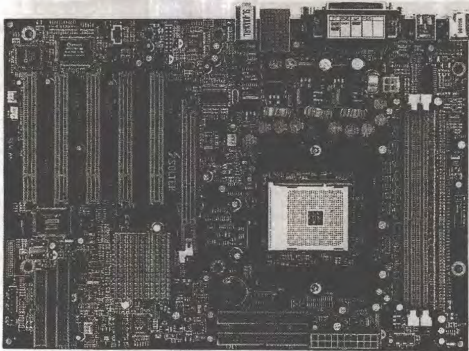
Рис. 4.19. Материнская плата Soltek K8AN-RL
