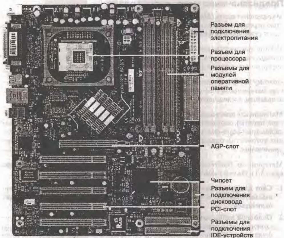
Рис. 4.1. Материнская плата
