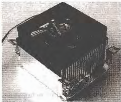
Рис. 5.16. Кулер Thermaltake P4 Volcano 478
