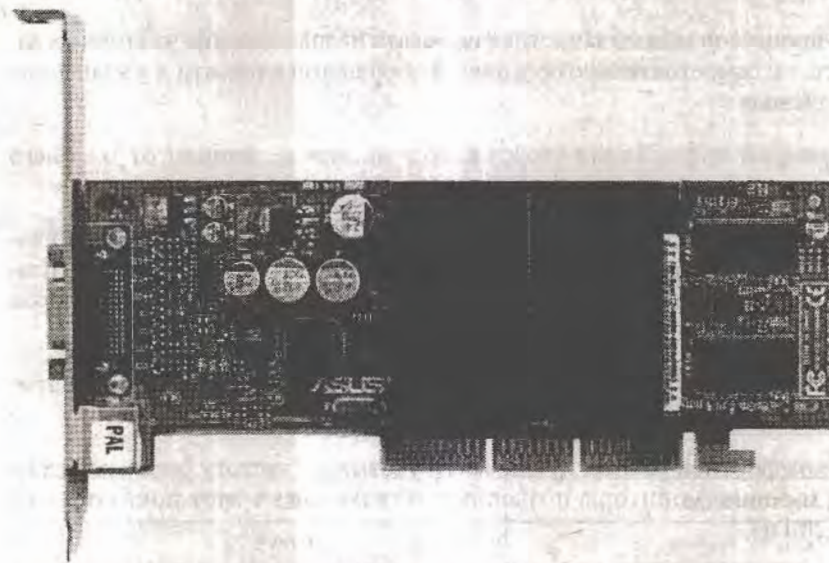
Рис. 7.1. Видеокарта на базе основного набора микросхем GeForce 4 MX440
