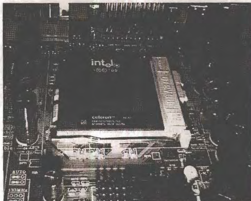
Рис. 20.5. Закрываем процессорный слот защелкой
