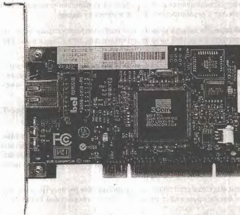
Рис. 13.1. Сетевая карта 3Com EtherLink XL 3C905C-TX-M
